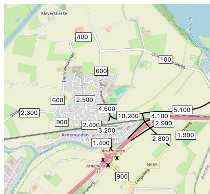
Figuur 3.10: Variant A3 verkeersintensiteiten
