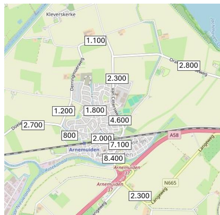
Figuur 3.19: Basisvariant B verkeersintensiteiten
