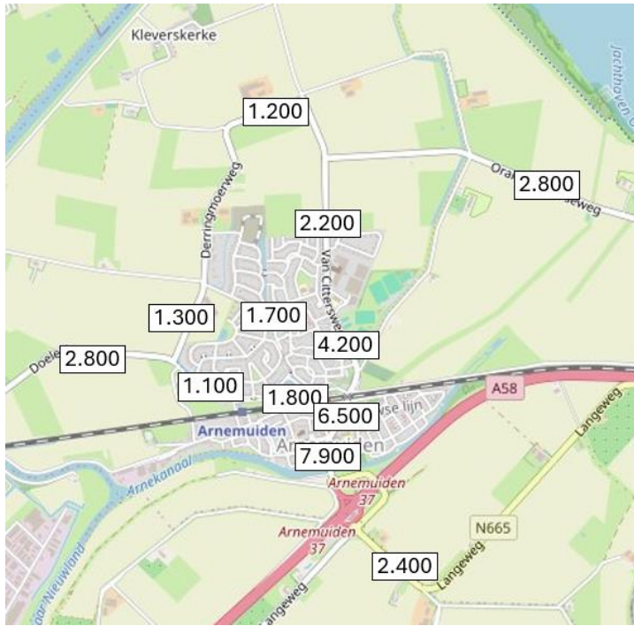
Figuur 3.24: Referentie 2030 verkeersintensiteiten
